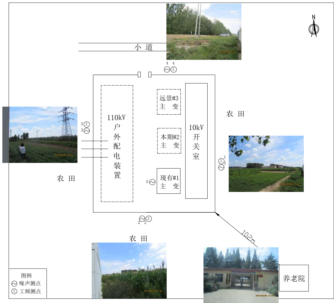
附图 2 110kV 洪庄变电站监测点位及周围环境示意图
