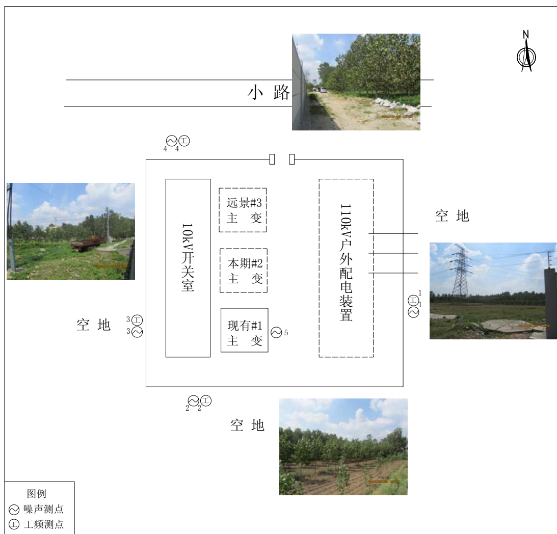
附图2 110kV 山左口变电站监测点位及周围环境示意图
