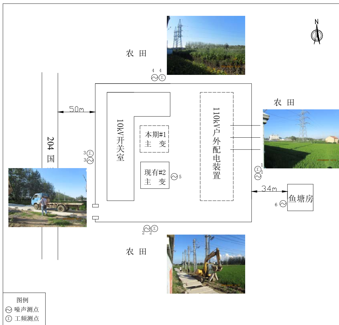
附图 2 110kV 墩尚变电站监测点位及周围环境示意图
