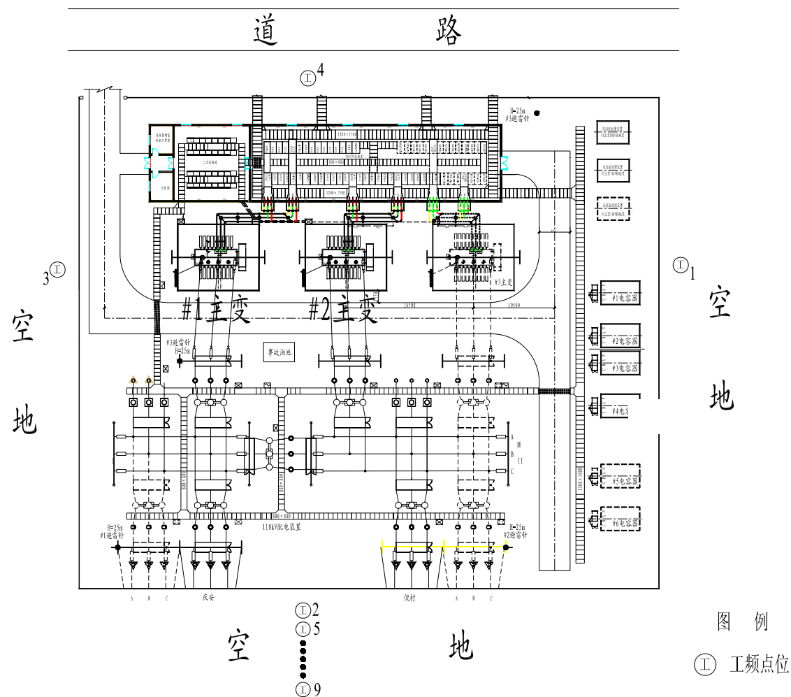
附图 4、110kV 联群变电站（类比站）监测点位示意图
