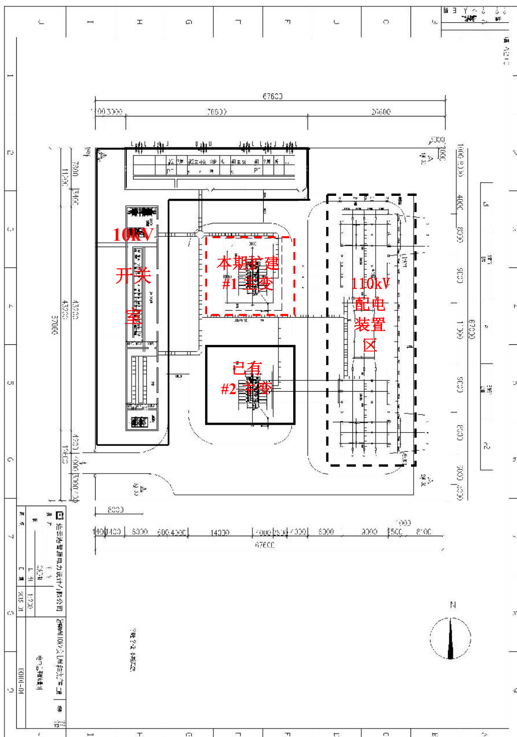
附图 3 110kV 墩尚变电站平面布置示意图
