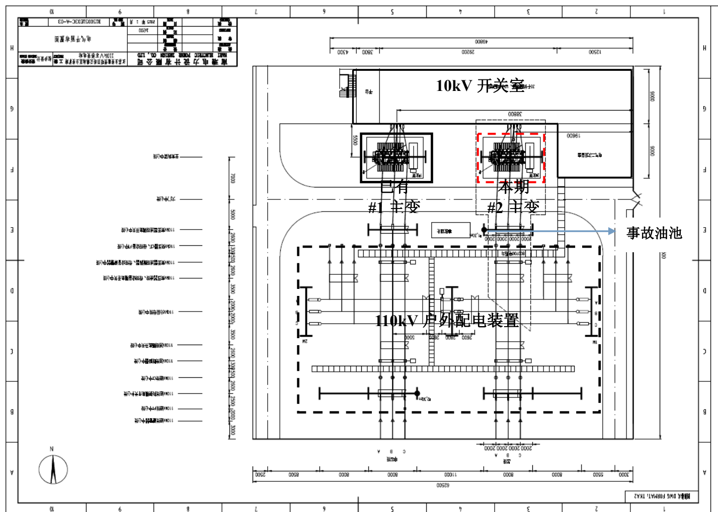
附图 3 110kV 石桥变电站平面布置示意图
