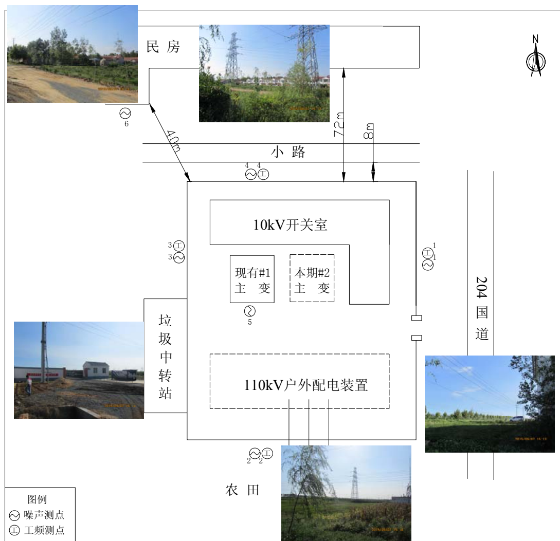
附图2 110kV 石桥变电站监测点位及周围环境示意图
