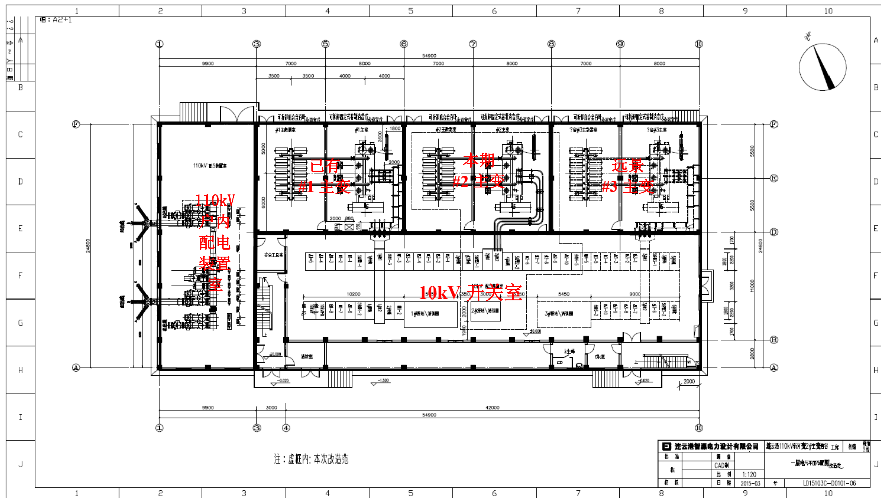
附图3 110kV 新河变电站平面布置示意图
