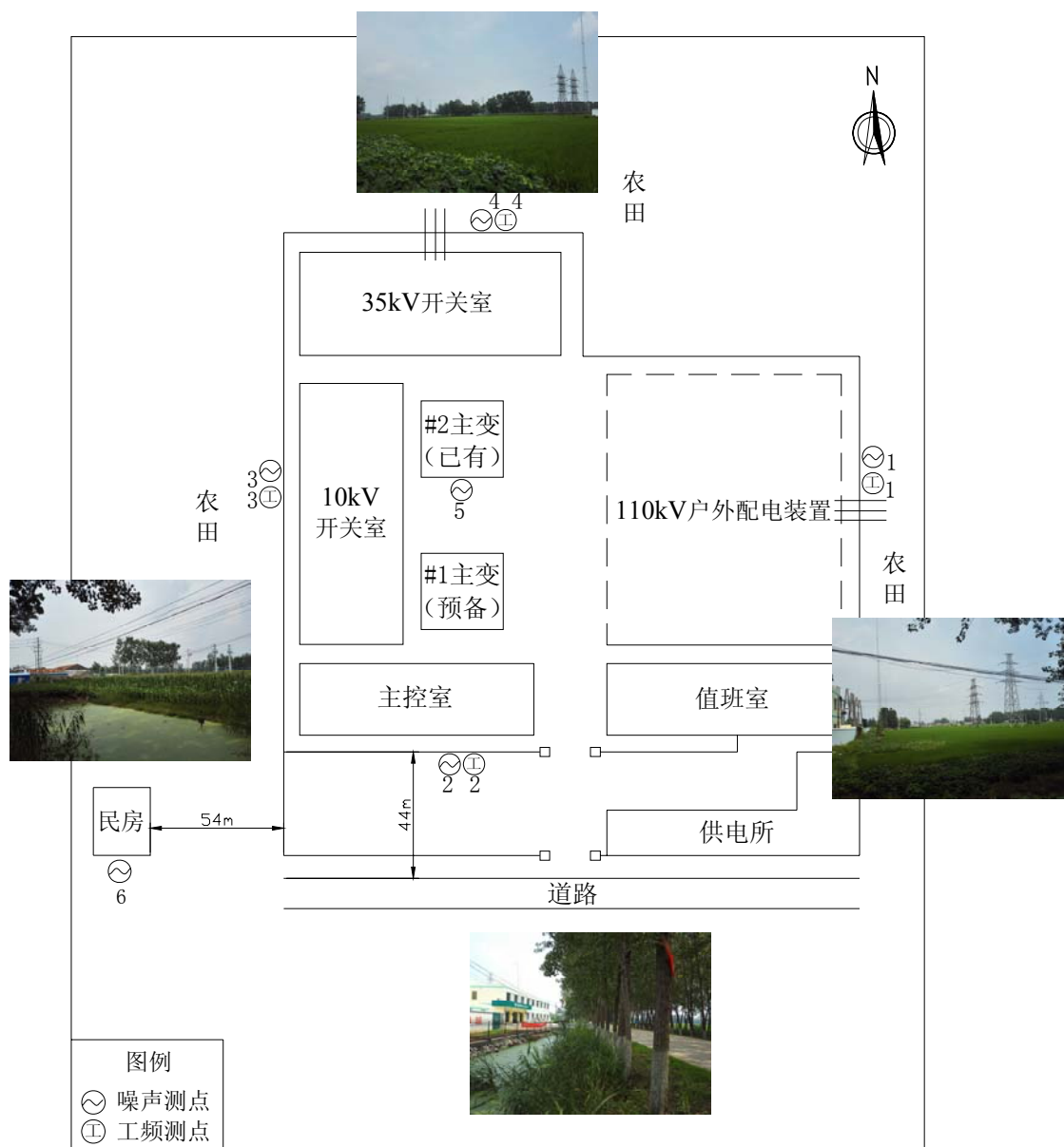
附图2 110kV三口变电站监测点位及周围环境示意图
