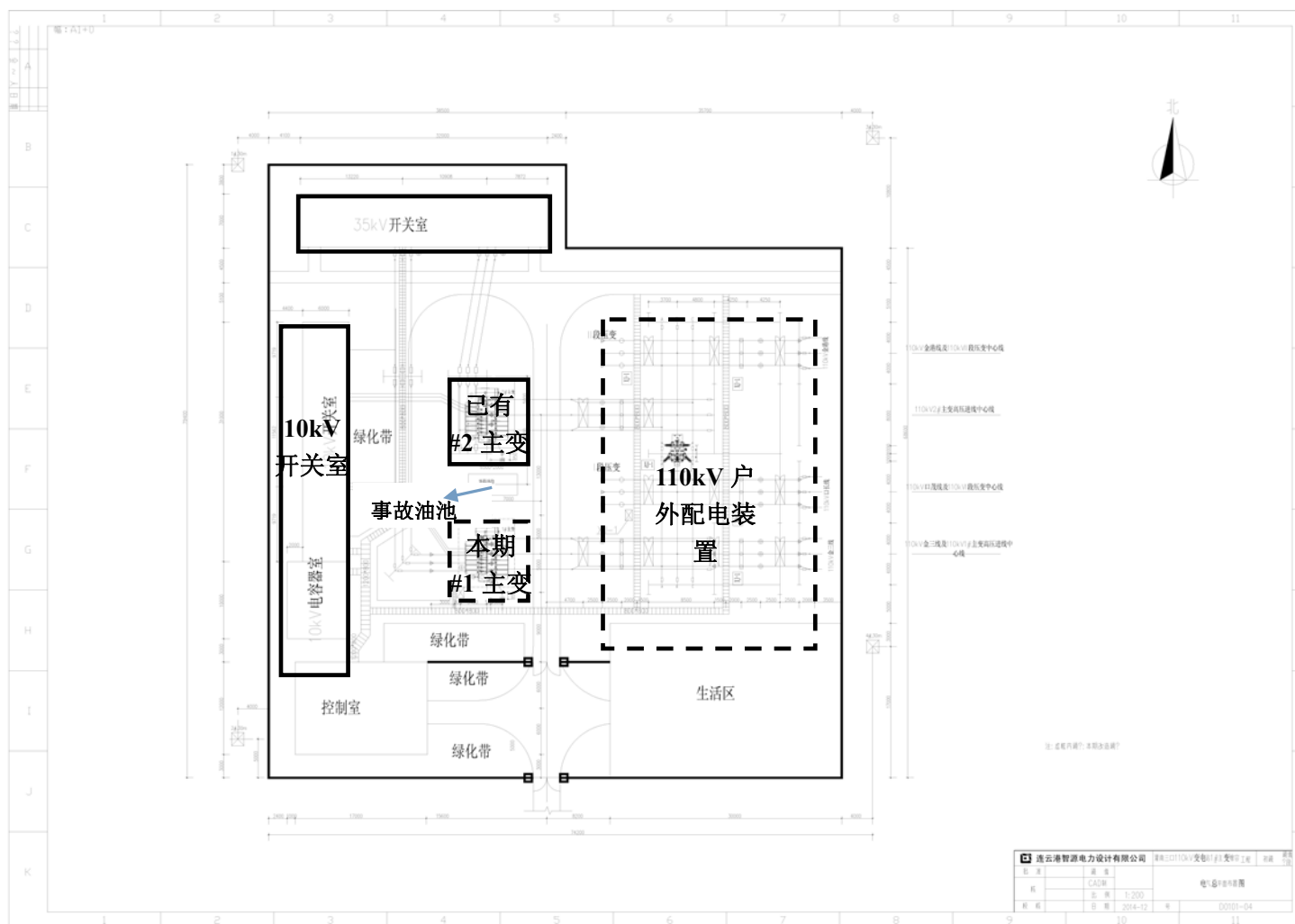
附图 3 110kV 三口变电站平面布置示意图
