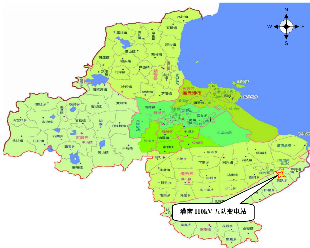
附图 1 灌南 110kV 五队变电站扩建#2 主变工程地理位置示意图
