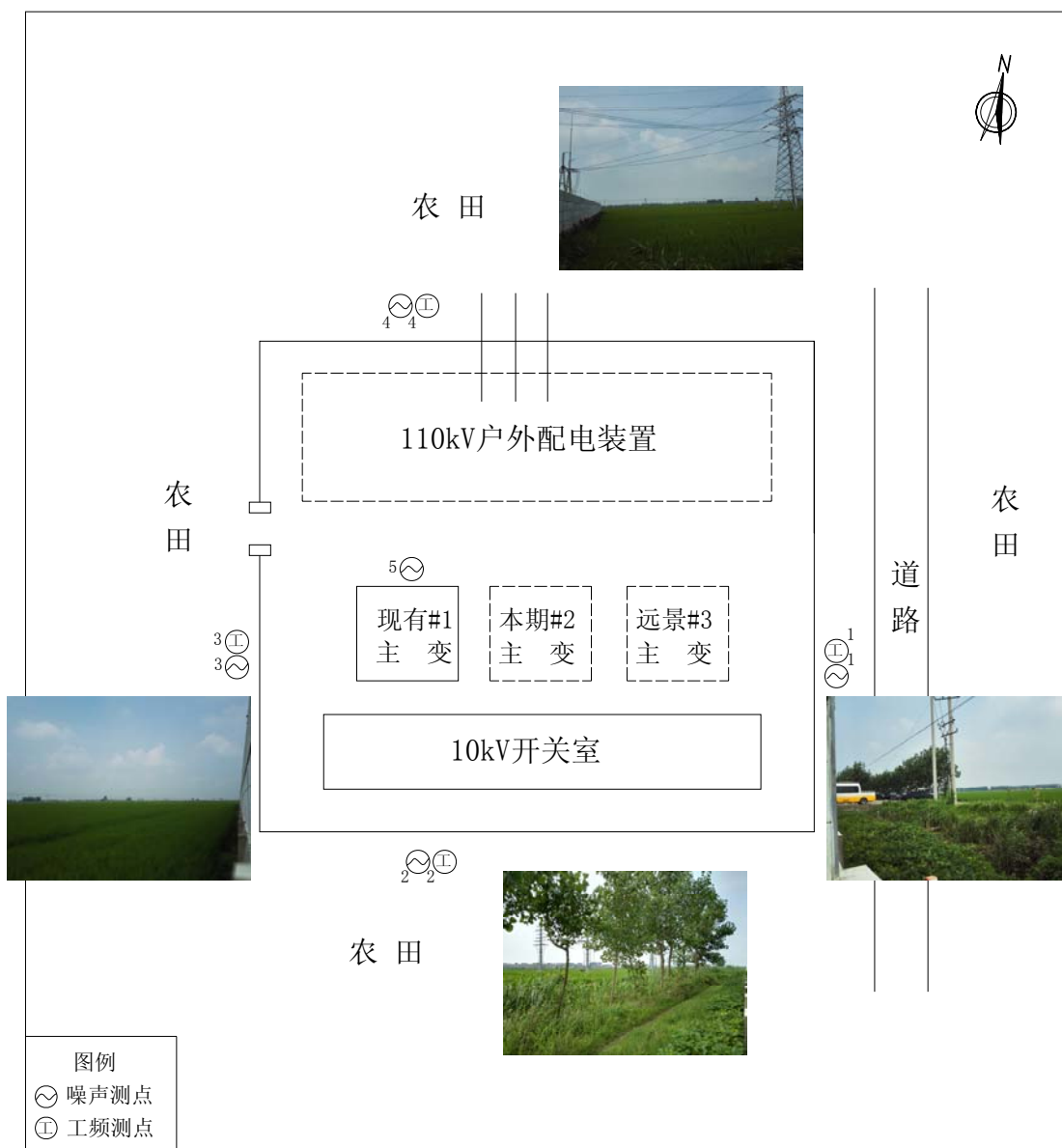
附图 2 110kV 五队变电站监测点位及周围环境示意图
