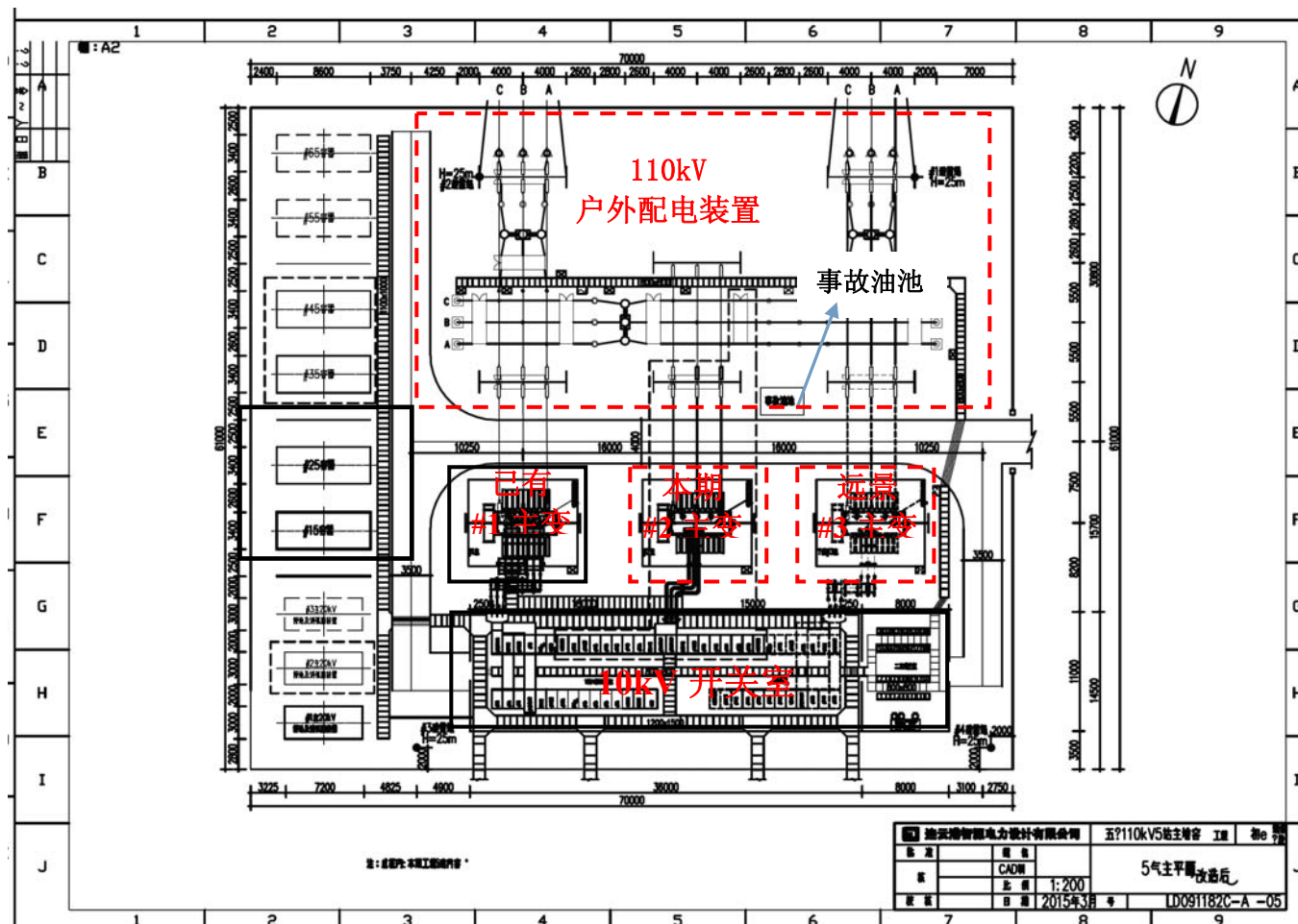
附图3 110kV 五队变电站平面布置示意图
