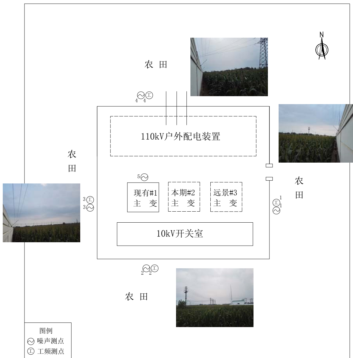
附图2 110kV 利华变电站监测点位及周围环境示意图
