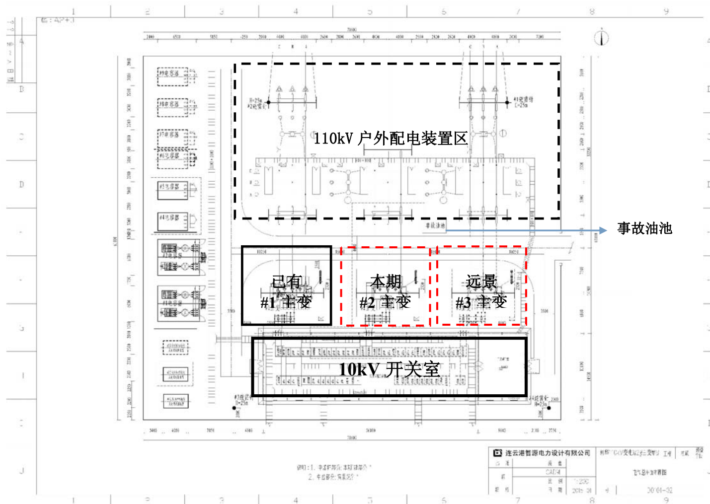
附图 3 110kV 利华变电站平面布置示意图
