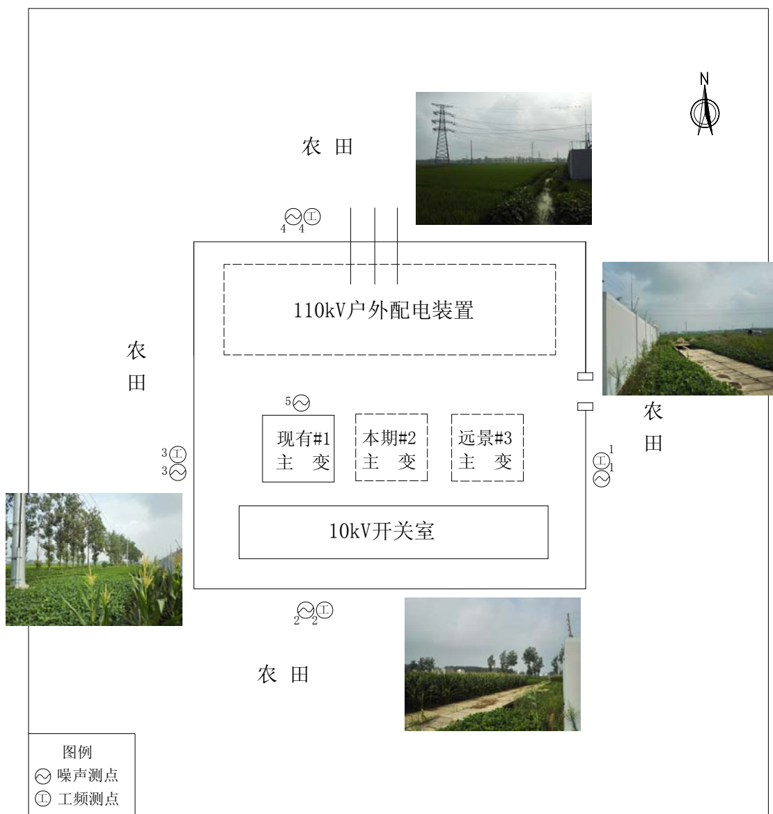
附图 2 110kV 盐东变电站监测点位及周围环境示意图
