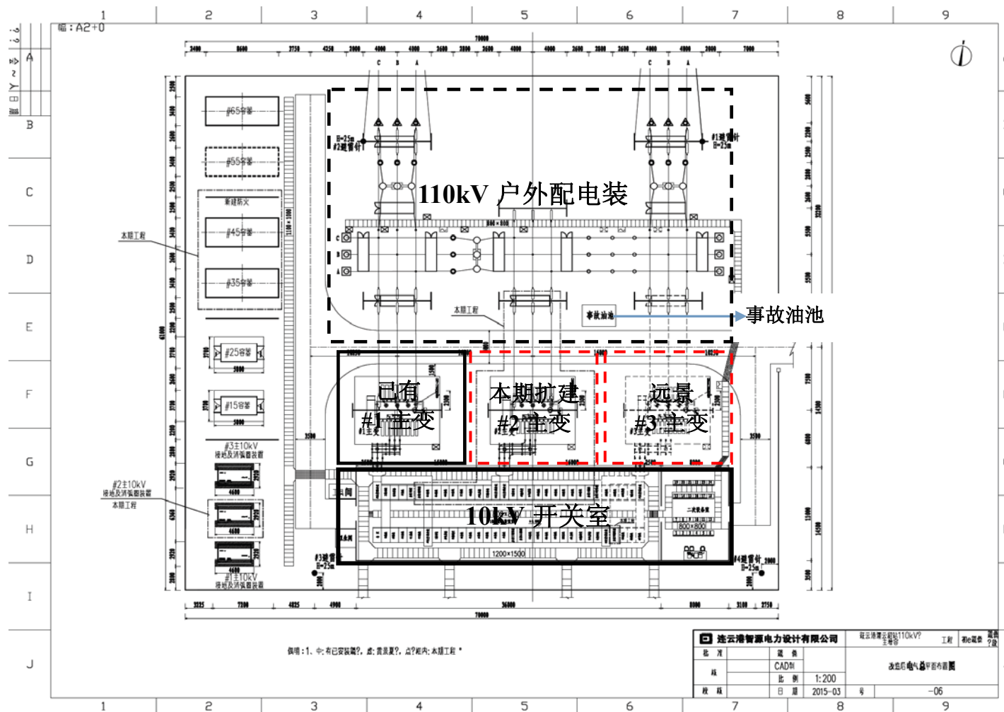
附图 3 110kV 盐东变电站平面布置示意图
