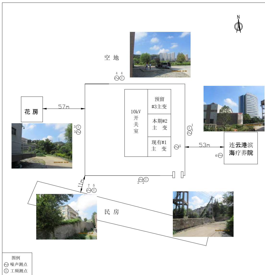
附图2 110kV 北崮变电站监测点位及周围环境示意图
