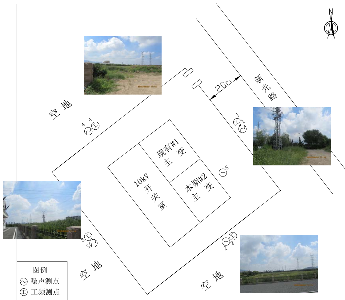
附图2 110kV 虎山变电站监测点位及周围环境示意图
