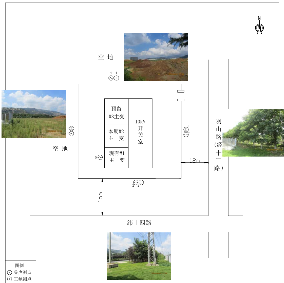
附图 2 110kV 羽山变电站监测点位及周围环境示意图
