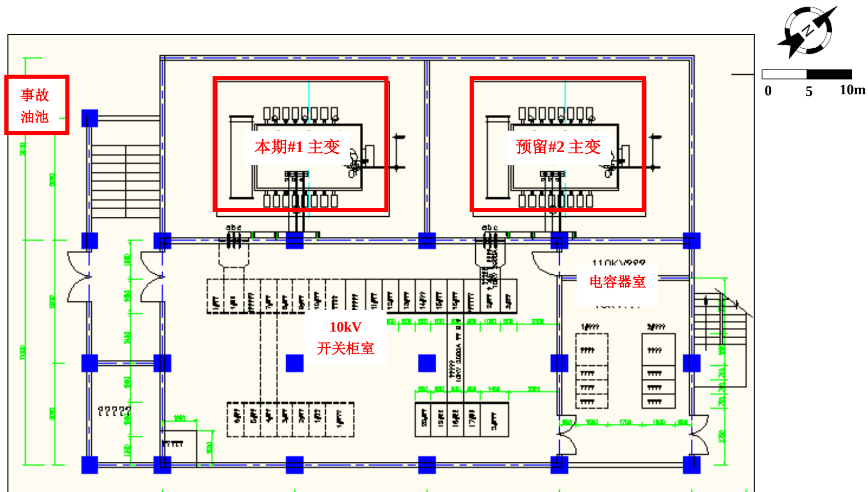
附图 4 110kV 利海化工变电站平面布置示意图
