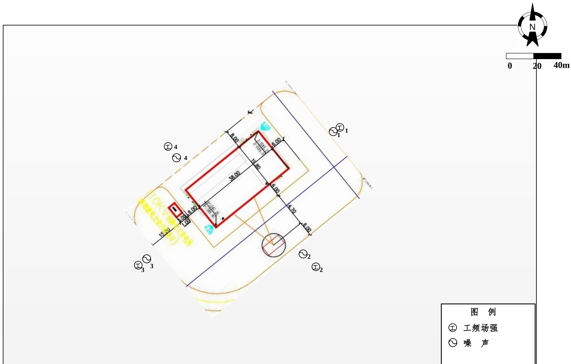
附图3 110kV 利海化工变电站监测点位及周围环境示意图
