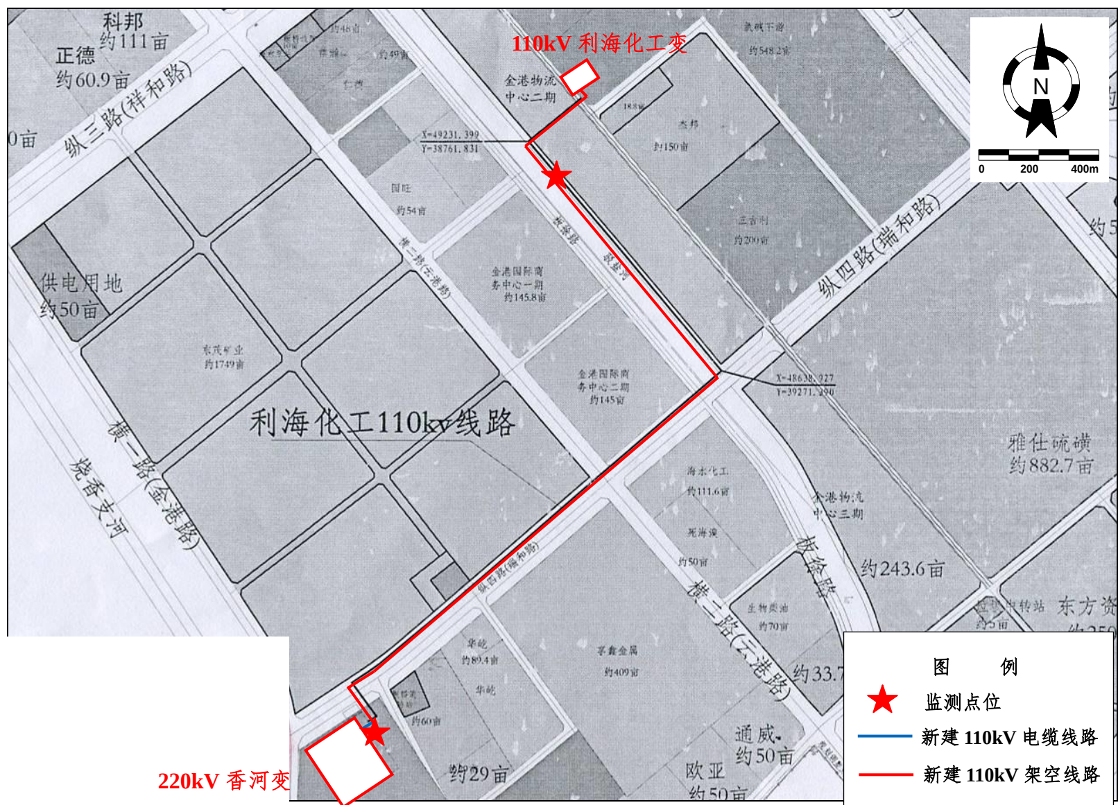
附图 5 110kV 香海 77D /香利 77C 线路径示意图
