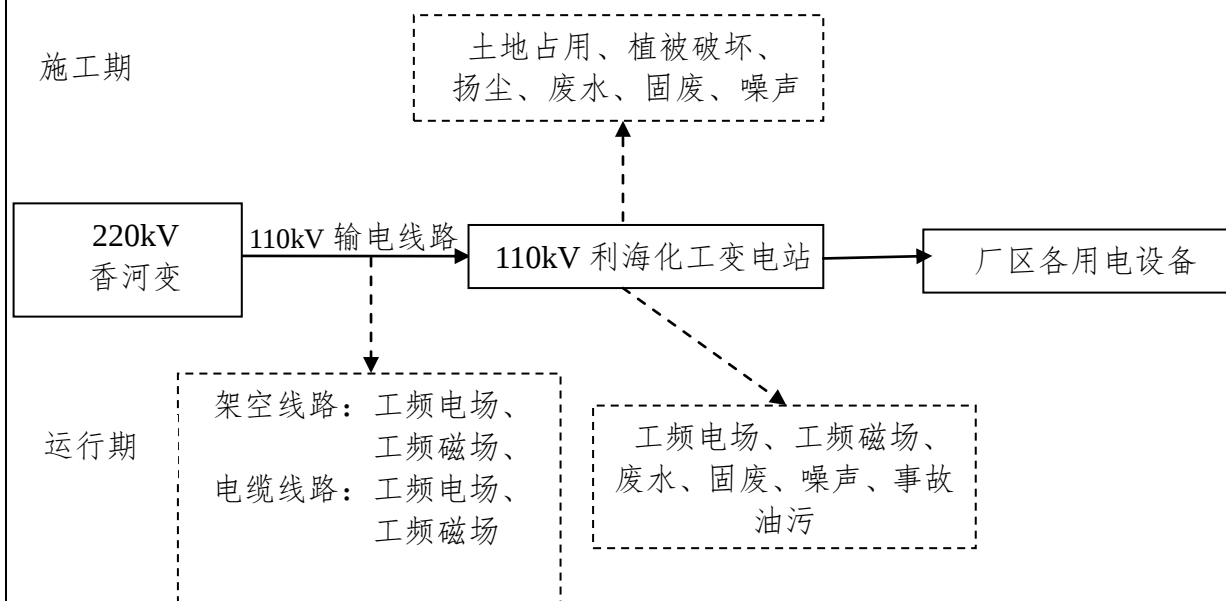
图 1 110kV 输变电工程运行期主要产污环节示意图
