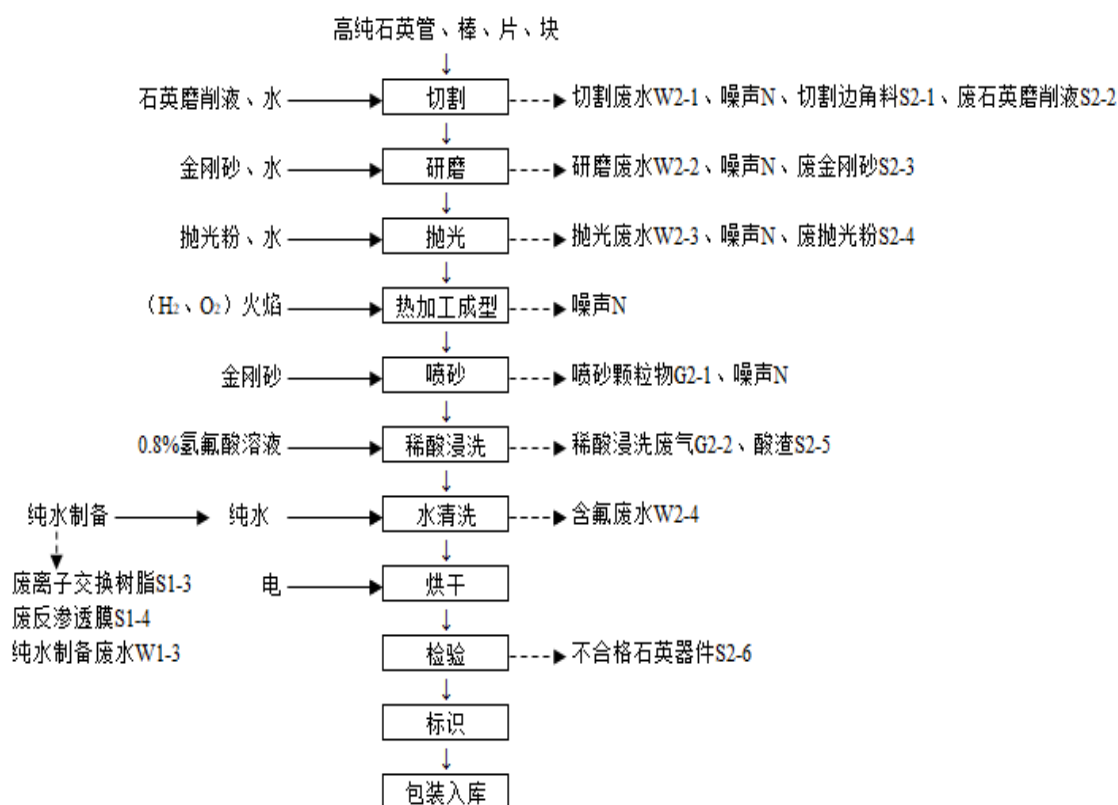
图2-2 工艺流程图
