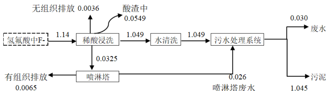
图2-2 本项目氟平衡 (t/a)
