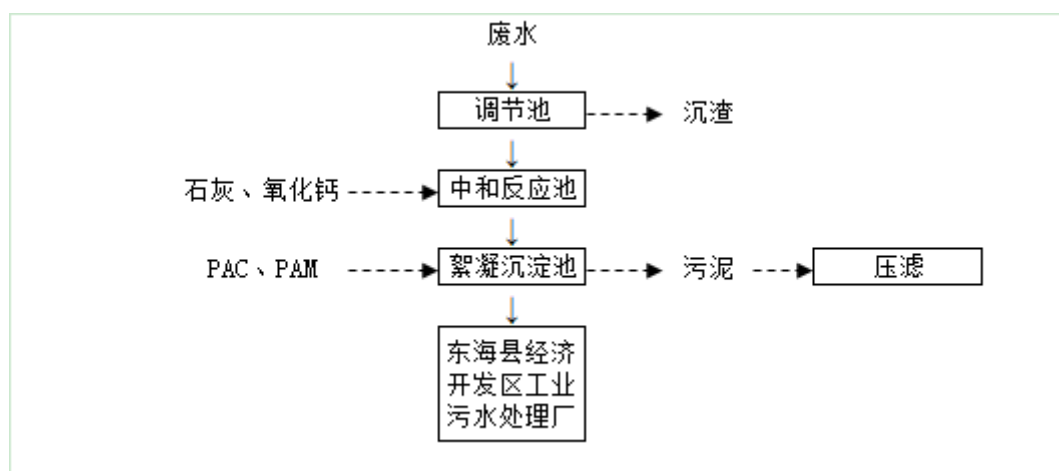
图4-1 本项目厂内污水处理系统处理工艺流程简图
