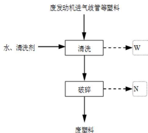
图 2-2 塑料零部件生产工艺及产污环节图
