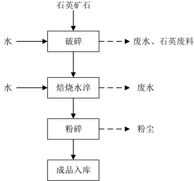
图 2-2 管类石英材料生产工艺及产污流程图
