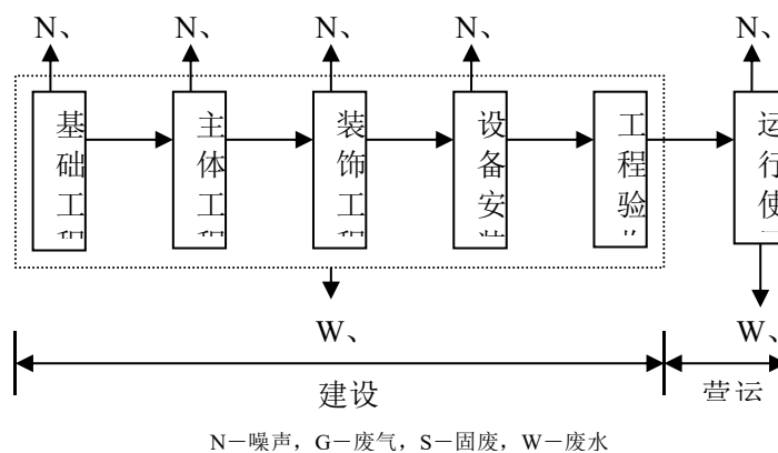
图 2-2 施工期工艺（或工作）流程图
