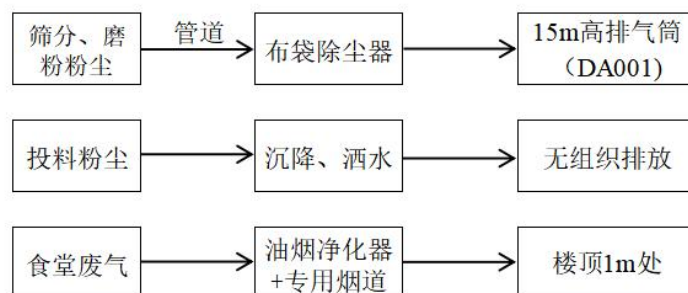
图4-1 本项目废气处理工艺流程
