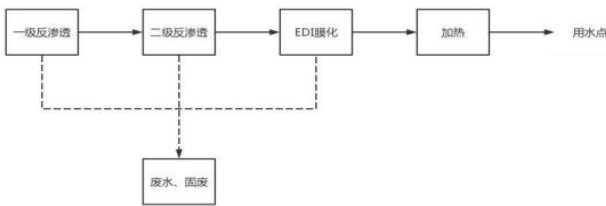
图 2-5 纯水制备工艺流程图
