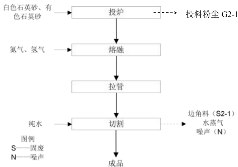
图 2-4 石英管生产线生产工艺流程图
