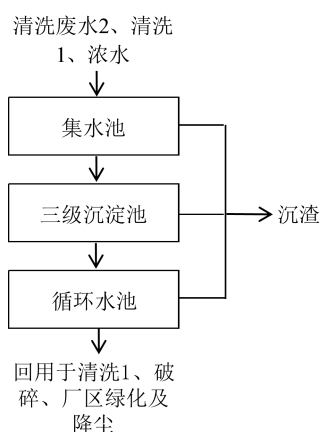
图 4-2 回用系统工艺流程图
