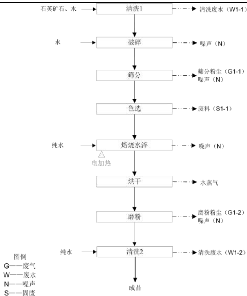
图 2-3 高纯石英砂生产线生产工艺流程图
