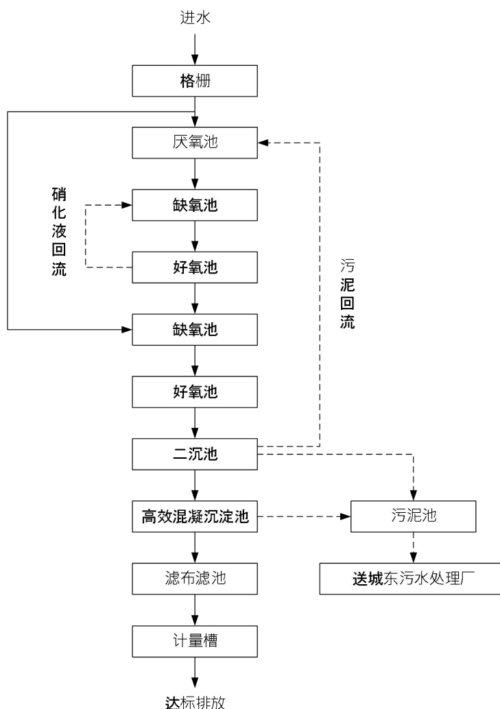
图 4-4 东海县山左口乡山西村生活污水处理厂处理工艺流程图
