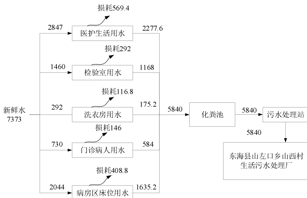
图 2-1 本项目水平衡图 (m 3 /a)
