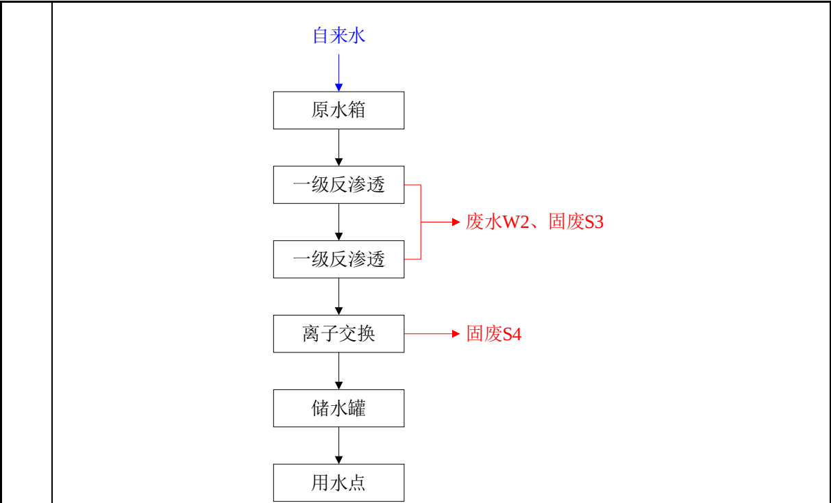
图2-3 纯水制备生产工艺流程及产污环节图
