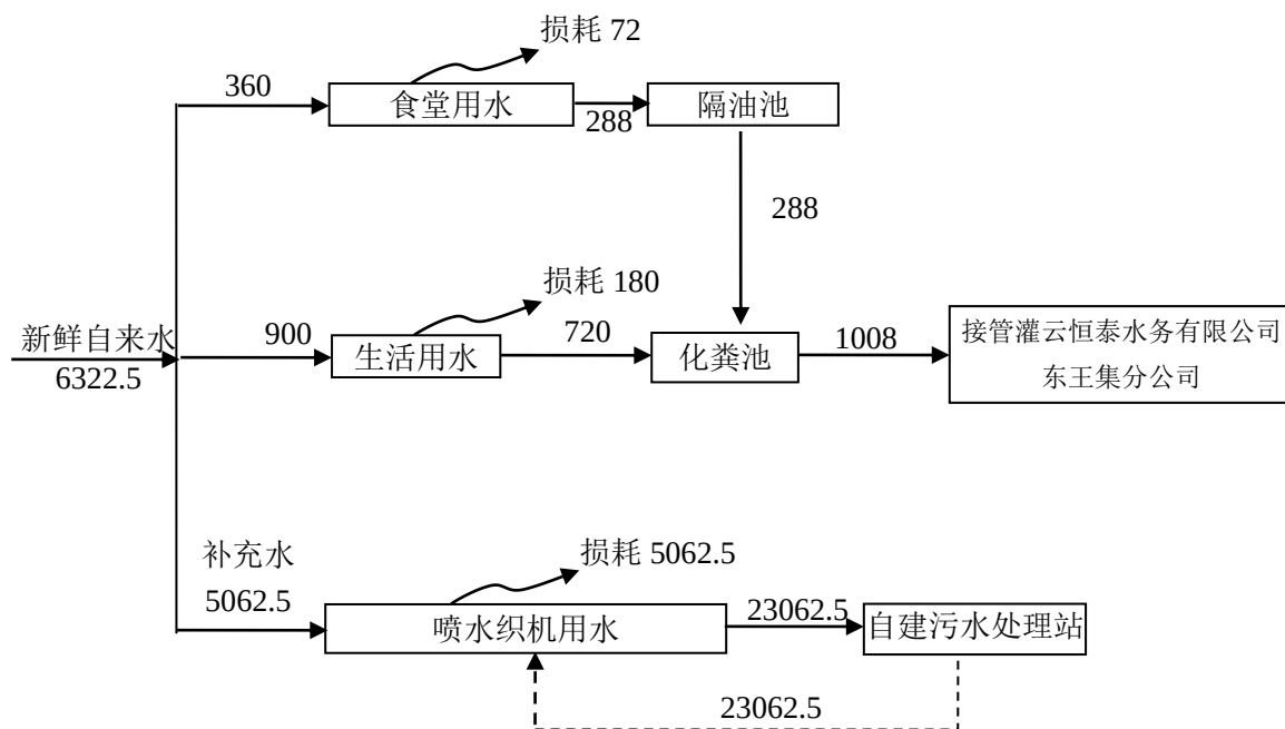
图 6.2-2 项目水平衡图 (单位: m 3 /a)
