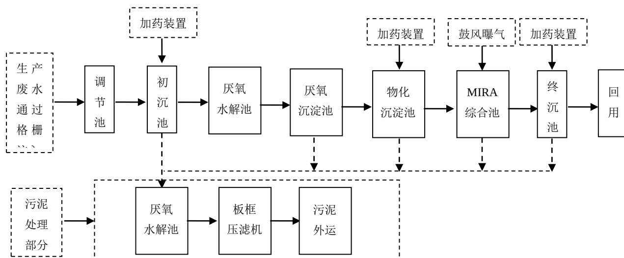
图 6.2-3 自建污水处理设施处理工艺图
